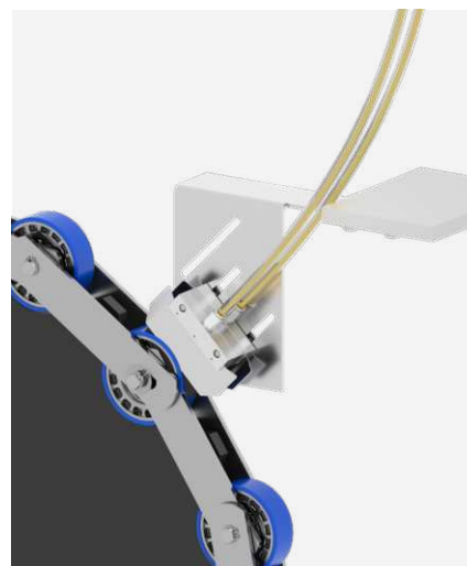
Lubrification de la chaîne des marches
