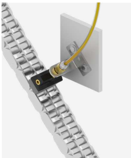
Lubrification de la chaîne d'entraînement
