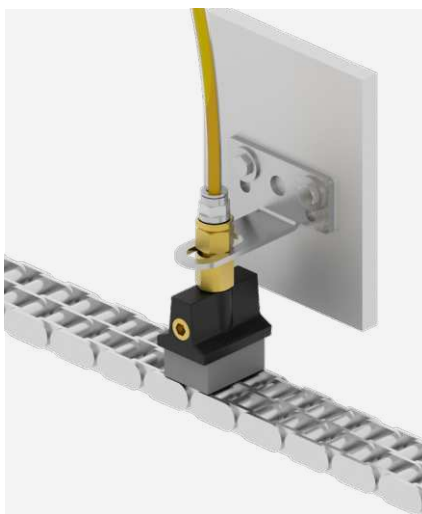
Lubrification de la chaîne de main courante
