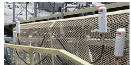
Indirekte Schmierung von Förderbandanlagen
