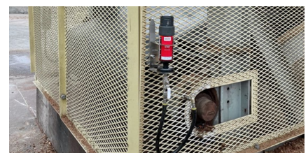
Lubricación de una cinta transportadora
