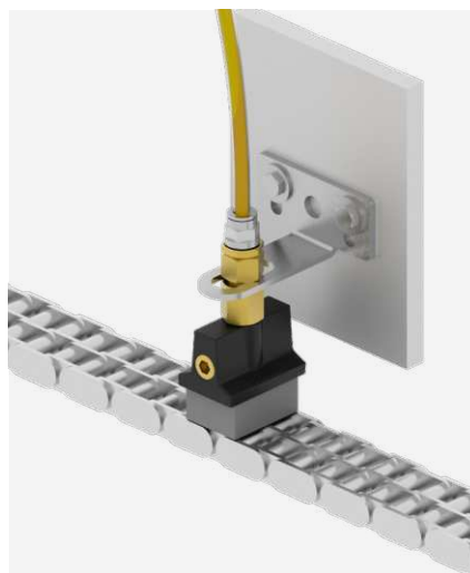
Lubrificazione della catena del corrimano
